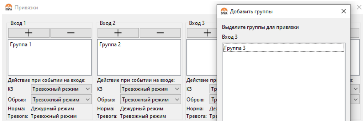
Рисунок 18 – Окно «Привязки». Настройка привязок групп светильников к тревожным входам
