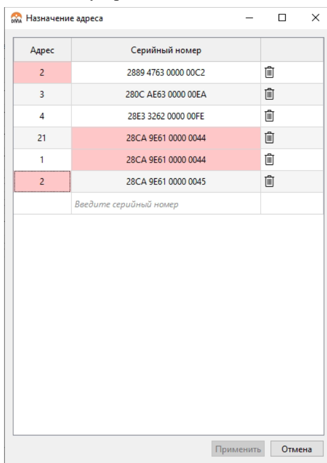
Рисунок 12 – Окно «Назначение адреса». Подсветка дубликатов значений
