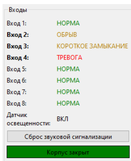
Рисунок 21 – Главное окно программы. Панель «Входы». Регистрация тревоги, обрыва и короткого замыкания. Включена звуковая сигнализация
