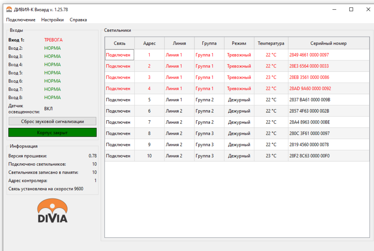
Рисунок 20 – Главное окно программы. Регистрация тревоги на тревожном входе 1. Корпус контроллера вскрыт. Звуковая сигнализация сброшена
