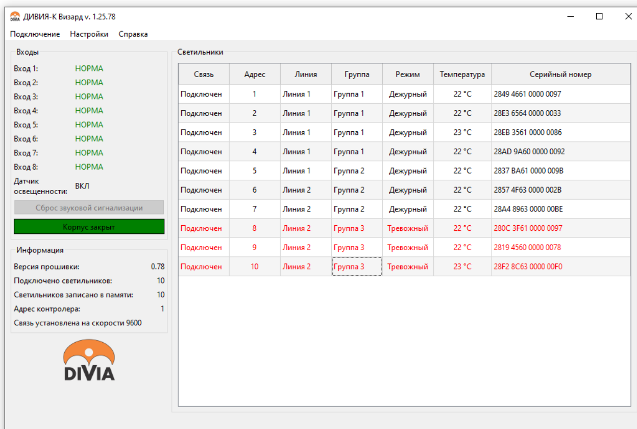
Рисунок 1 – Основное окно программы
