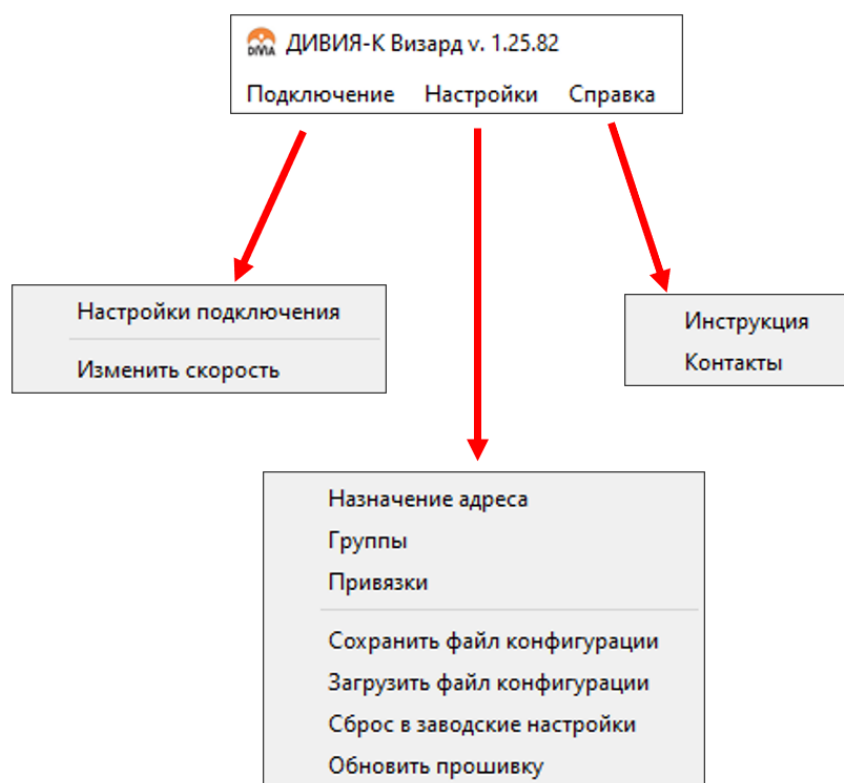
Рисунок 2 – Главное меню программы
