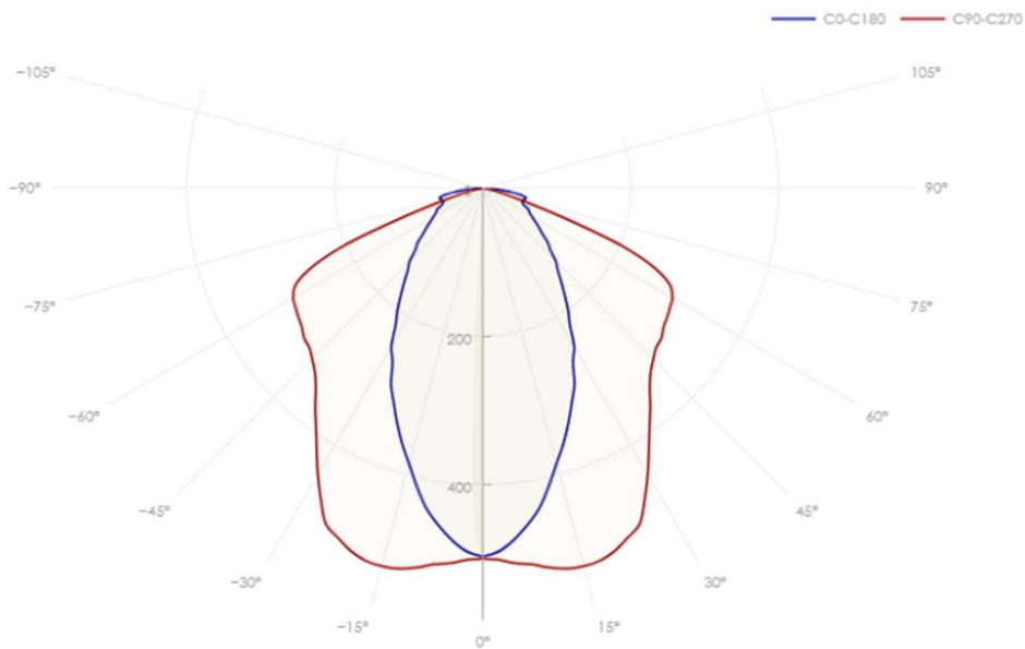
Рисунок 2 – Кривая силы света «Д»
