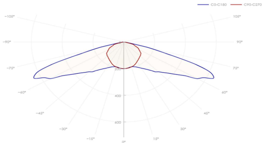
Рисунок 1 – Кривая силы света «Ш1-1»
